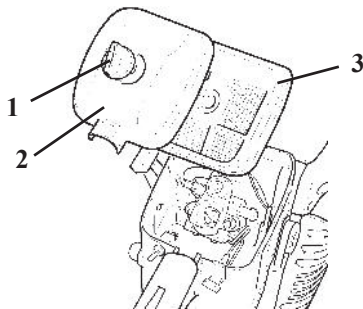
KRAFTSTOFF-FILTER Bild 1
