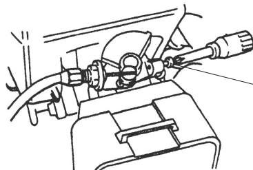
Idle Speed Adjustment Screw/ Tornillo de ajuste del ralenti/ Parafuso do ajustador da velocidade ao ralenti
